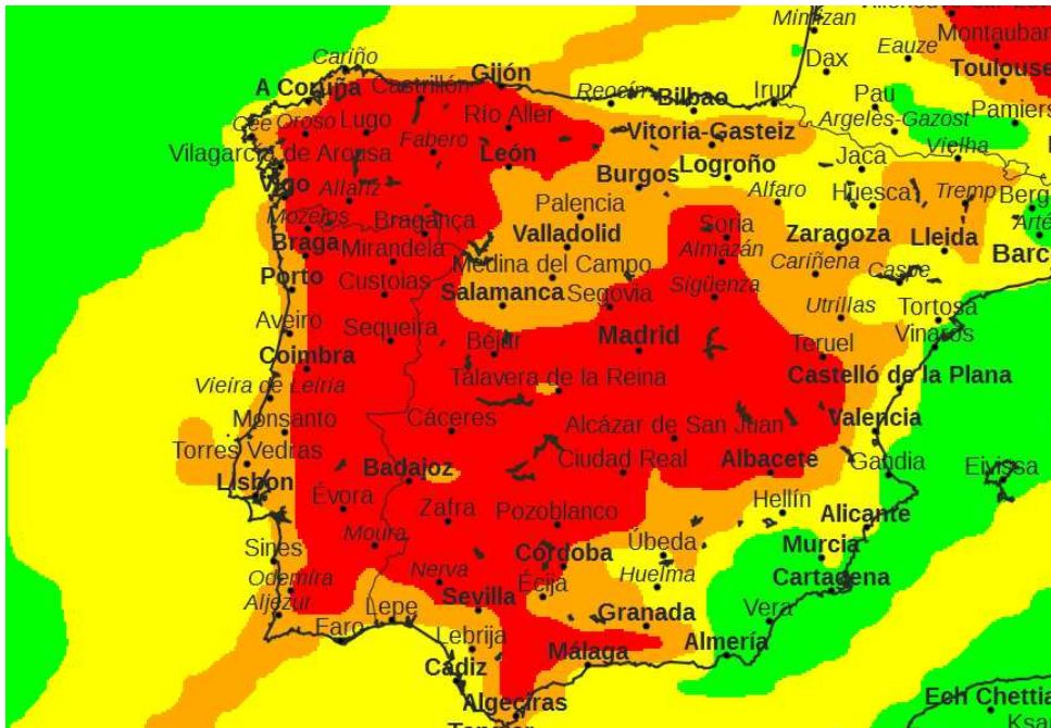
Figura 4 - Risco de formação de nevoeiro.
