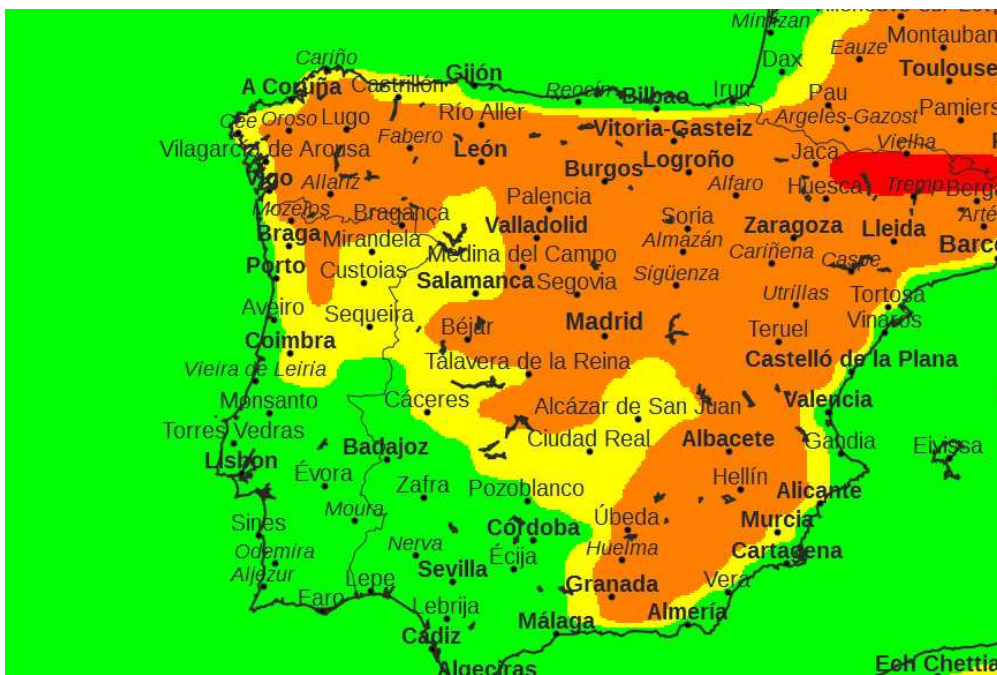
Figura 5 – temperatura.
