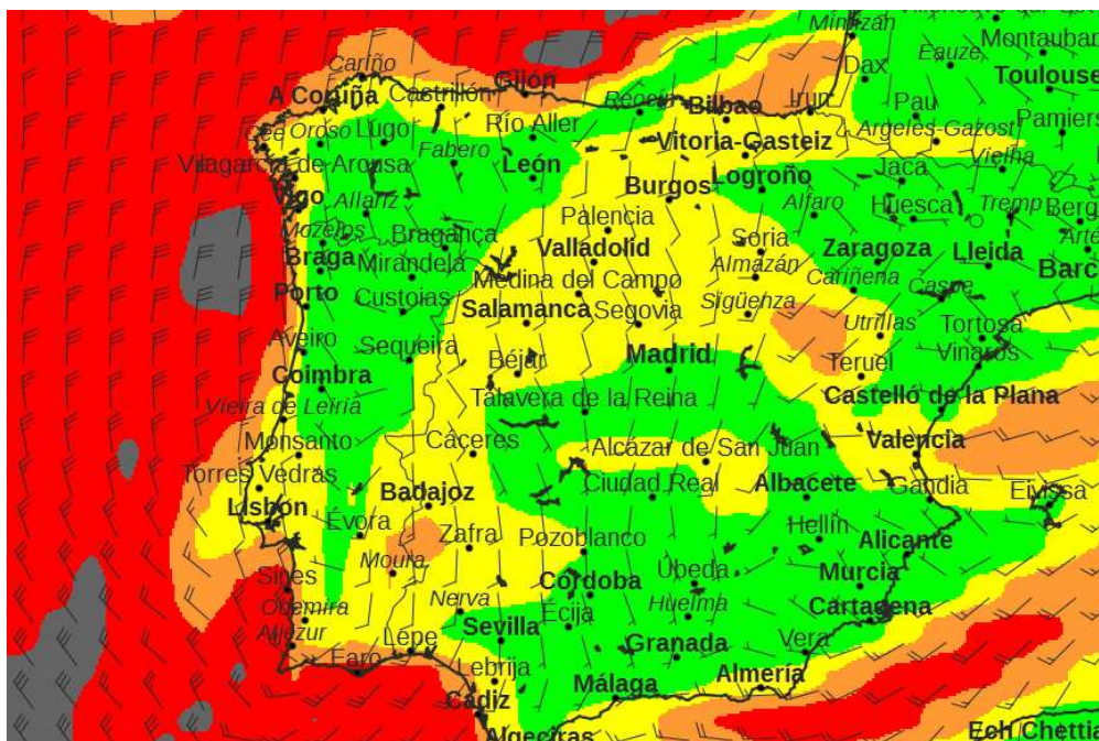
Figura 1 - Vento – direção e intensidade.
