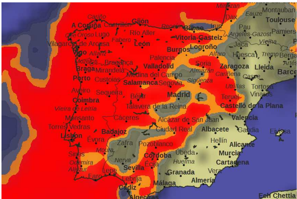
Figura 3 – Nebulosidade.
