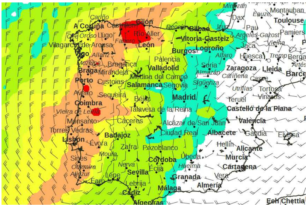
Figura 2 - Precipitação – Intensidade (esta apresenta-se com a direção e intensidade do vento).
